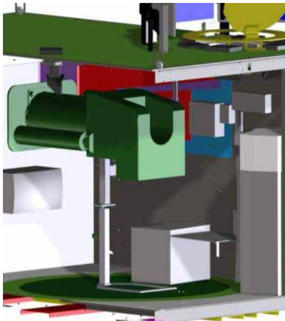
Simulation du canon. À l'intérieur du bloc culasse, se trouve le mécanisme pressurisé qui devra être actionné par le chargeur lorsqu'il simule le chargement d'un obus.
