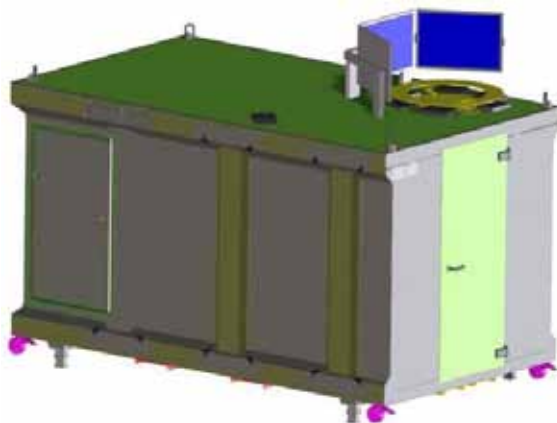
Vue extérieure du simulateur. Porte d'entrée à l'arrière, panneau de maintenance des ordinateurs sur le côté et écrans 24 pouces pour la vision tête sortie du CC de 120 degrés.
