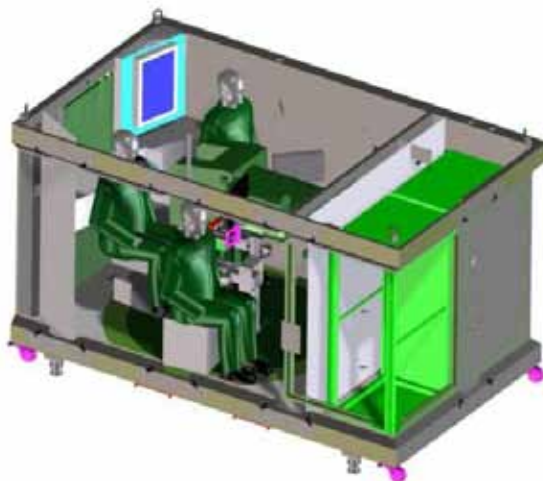
Modèle de disposition intérieur du simulateur. Notez en bleu du côté chargeur l'écran tactile qui remplacera le compartiment de munitions.
